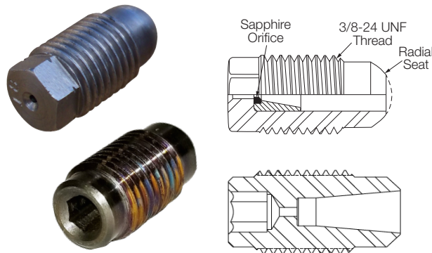
FOUR UHPX/UHPXi/UHPXD NOZZLES
