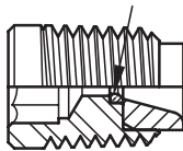
Sapphire Orifice
